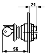
Tête de bouton-poussoir à frapper "ARRET D'URGENCE" avec clé
