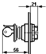
Schlagastervorsatz "NOT-AUS" mit Schlüsselentriegelung
