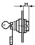
Tête de bouton-poussoir à clé
