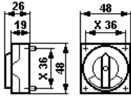
Tête de commutateur de commande Ex 23
