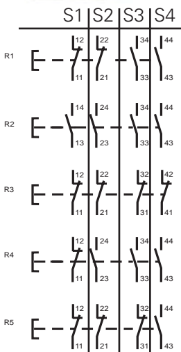
Actuator 2 x 2 pole
