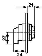
Tête de commutateur de commande et de potentiomètre *1
